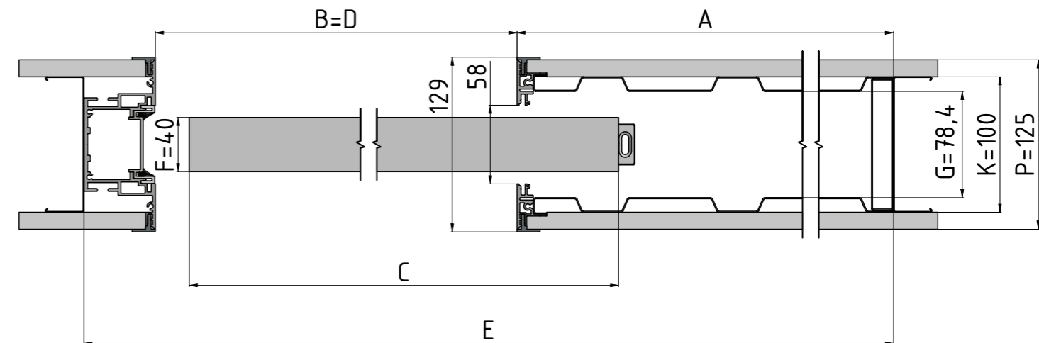
Horizontální řez pouzdrém EMOTIVE II STANDARD s dřevěným dveřním křídlem tloušťky 40 mm.
